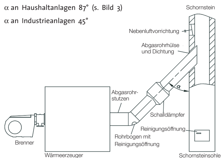
Bild 1: Komponenten einer Abgasanlage
