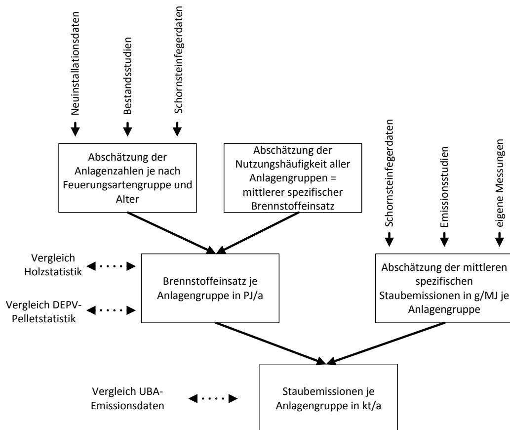
Abbildung 1: Methodisches Vorgehen bei der Abschätzung von Brennstoffeinsatz und Staubemissionen in dieser Studie
