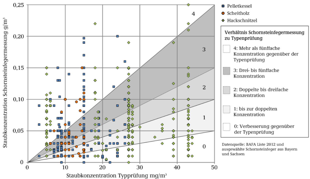
Abbildung 2: Vergleich von Staubemissionswerten zwischen Typenprüfergebnissen und für die gleichen Anlagen von Schornsteinfegern gemessenen Staubemissionen
